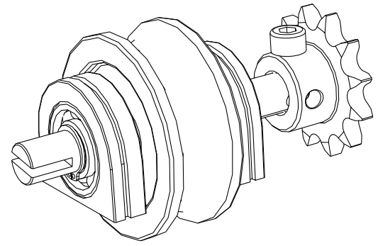
Ролик приводной
